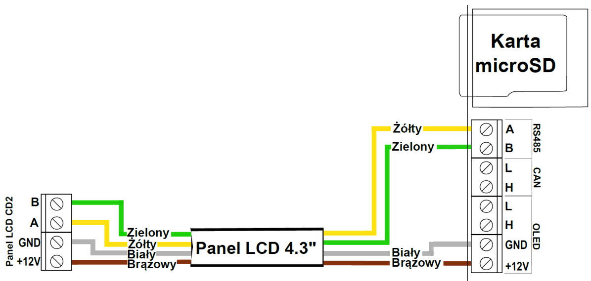
Ilustracja 1: Wyprowadzenia wtyczki przewodu do panelu CD2 4.3"
